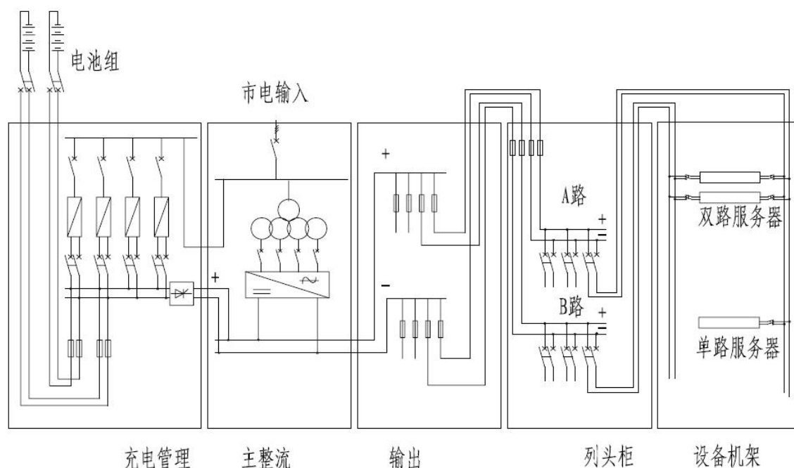
图A.1 二级配电结构示意图
