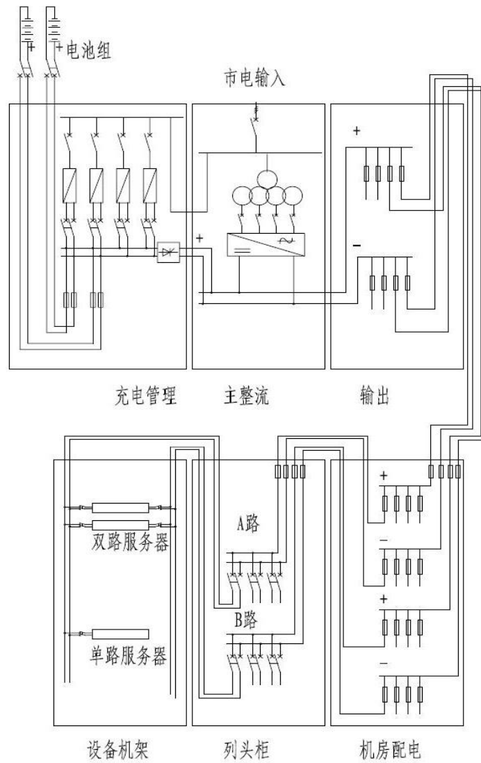
图A.2 三级配电结构示意图
