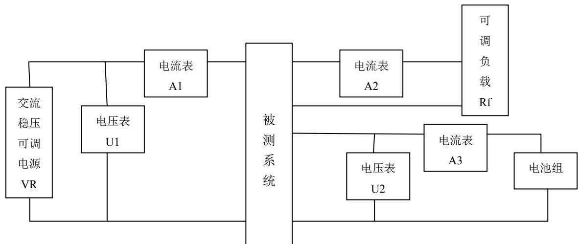
图1 系统测试基本原理图
