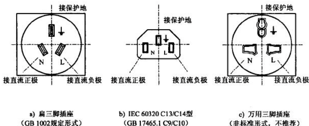
图A.4 设备机架内插座接线示意图
