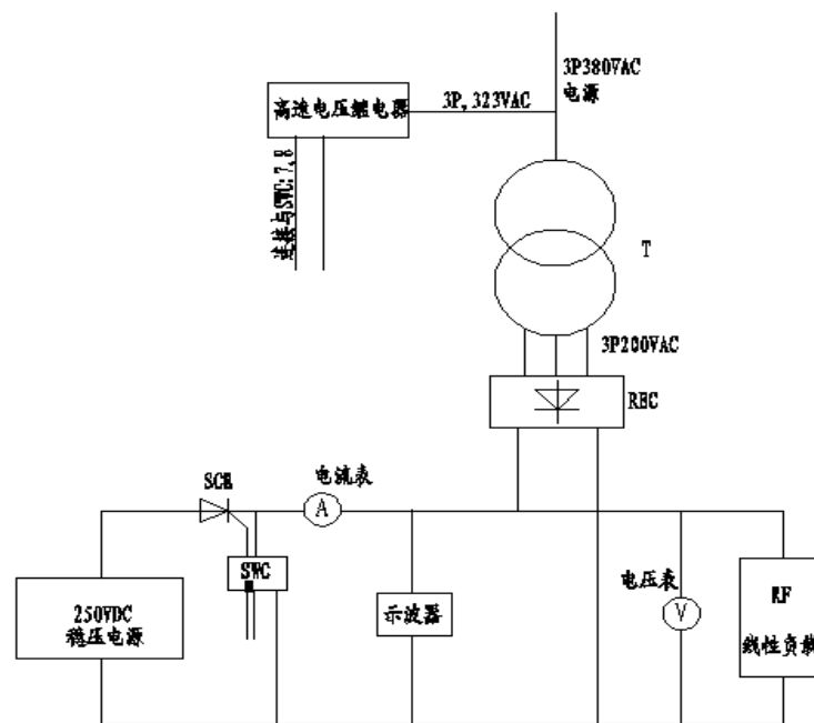
图4 静态开关测试原理图
