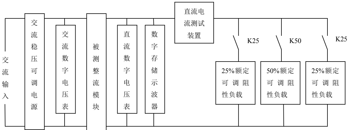
图3 负载效应恢复时间（动态响应）试验电路
