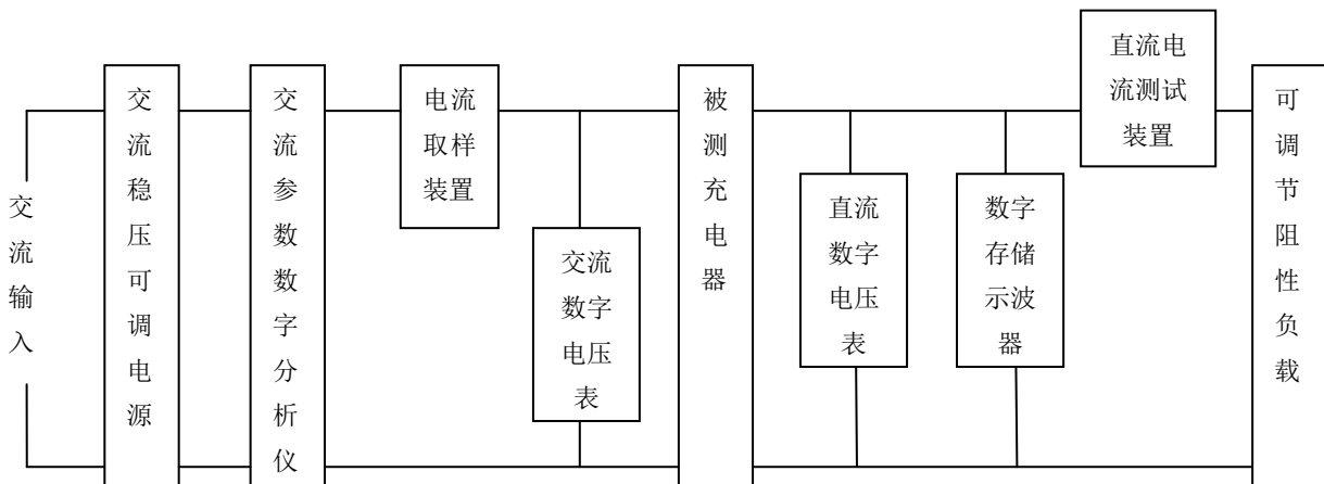
图2 充电模块测试基本原理图
