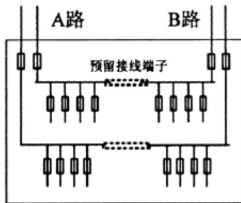
图A.3 双路改单路示意图
